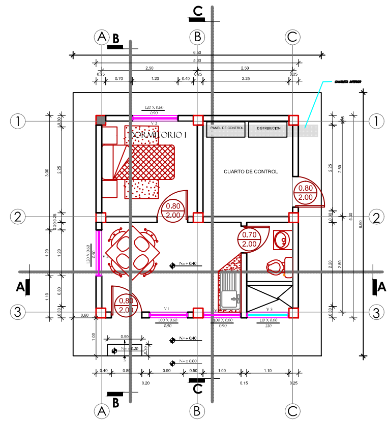
PLANTA NIVEL +0.40 ESC. 1:50
